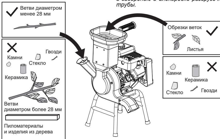
Рис. 11 Разрешенные и запрещенные для измельчения материалы
