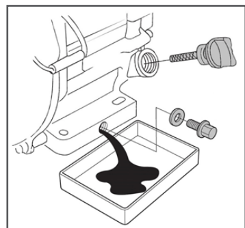
Рис. 12 Замена моторного масла
