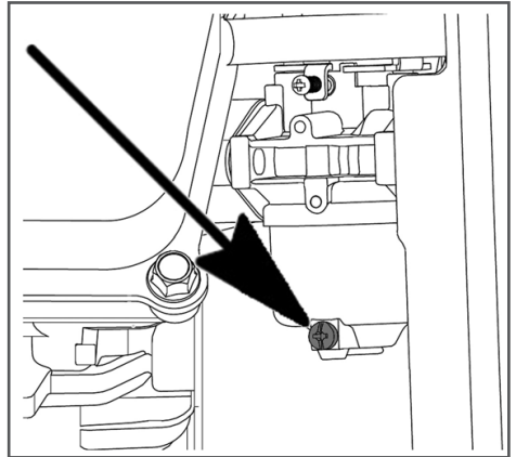
Рис. 16 Слив топлива с поплавковой камеры карбюратора
